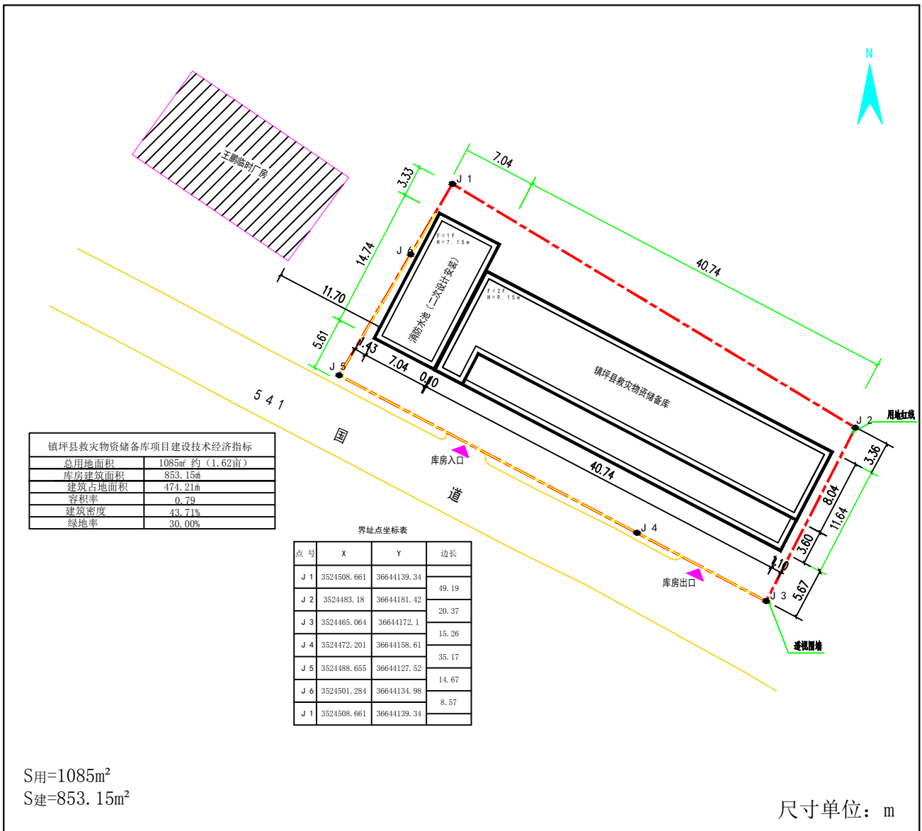
镇坪县救灾物资储备库项目总平面图
