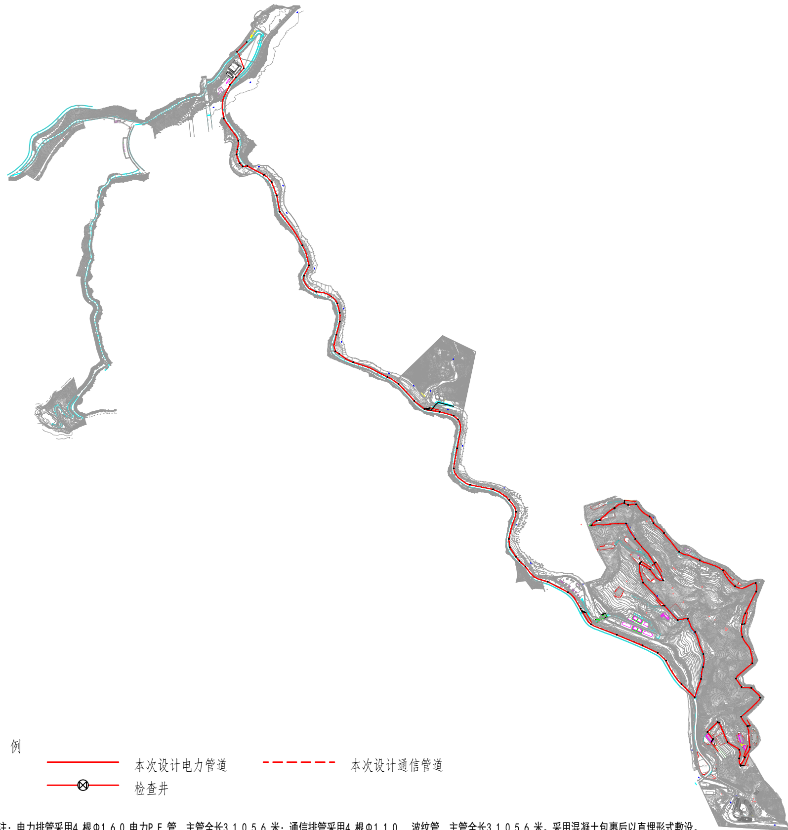
附图1：电力、通信总平面布置图
